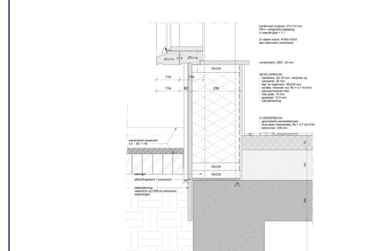
Afbeelding 6, 7, 8. Linksboven: dwarsdoorsnede met links de belending en rechts de gevel aan het kerkplein voor de Laurentiuskerk. Linksonder: horizontaal detail met zinken bekleding tegen de steunbeer van de Laurentiuskerk, verspringende smalle en brede kozijnen, dubbele kolommen en de vooruitspringende entree. Rechts: verticale details van de luifel met daarboven zinken gevelbekleding met luifel en plafond op zelfde hoogte en onderdetail van het kozijn met brede vensterbank op een hardstenen plint 2025.
