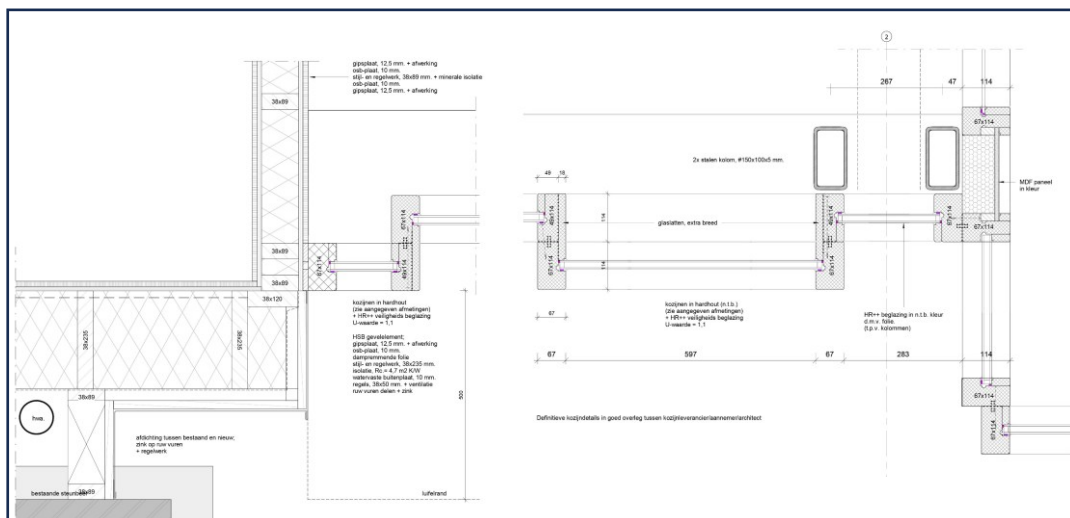
Afbeelding 6, 7, 8. Linksboven: dwarsdoorsnede met links de belending en rechts de gevel aan het kerkplein voor de Laurentiuskerk. Linksonder: horizontaal detail met zinken bekleding tegen de steunbeer van de Laurentiuskerk, verspringende smalle en brede kozijnen, dubbele kolommen en de vooruitspringende entree. Rechts: verticale details van de luifel met daarboven zinken gevelbekleding met luifel en plafond op zelfde hoogte en onderdetail van het kozijn met brede vensterbank op een hardstenen plint 2025.
