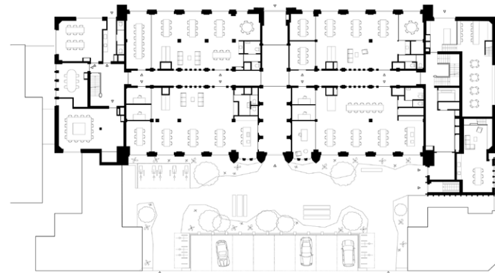
begane grond
