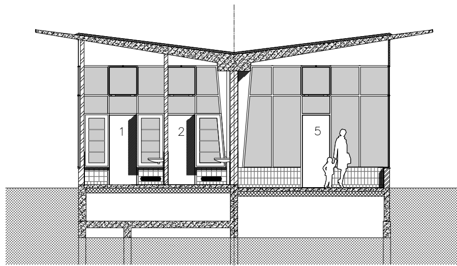
doorsnede Dd
