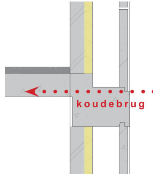
oorspronkelijk vloerranddetail (boven) en voorgesteld (onder)
