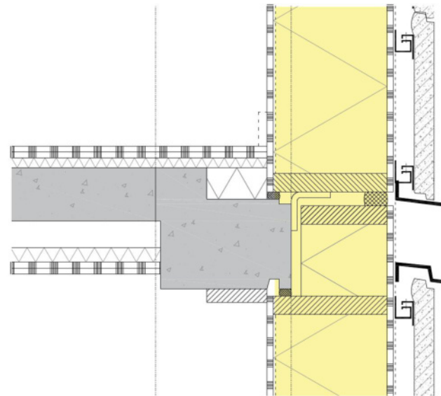
oorspronkelijk vloerranddetail (boven) en voorgesteld (onder)
